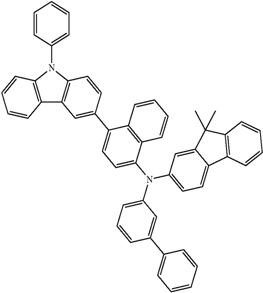
HT10
