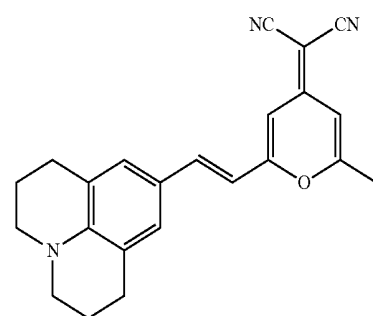
DCM
